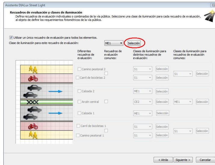
Ilustración 382 Recuadros de evaluación y clases de iluminación
